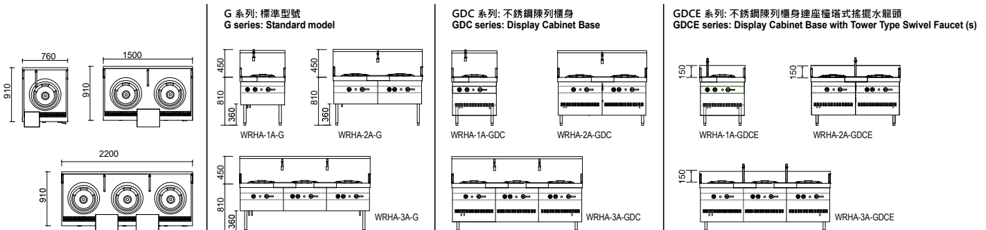
Ø75mm 強力溝風爐頭 Ø75mm Air blast burner assembly
